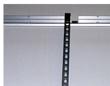
Hängstolpe och väggskena
